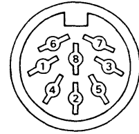
ACC(1) 後面パネルから見た図
