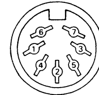
ACC(2) 後面パネルから見た図
